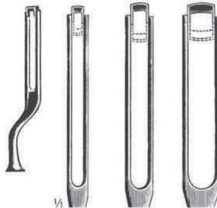
STI-21-7205 3 mm STI-21-7206 4 mm STI-21-7207 5 mm
